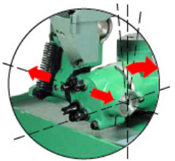
Seitliche Kopf-Verstellmöglichkeit für Schnitte 45° senkrecht nach links und Längsschnitte.
