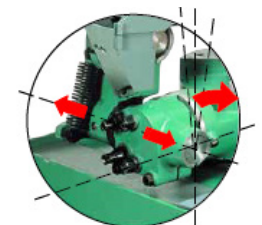
Seitliche Kopf-Verstellmöglichkeit für Schnitte 45° senkrecht nach links und Längsschnitte.
